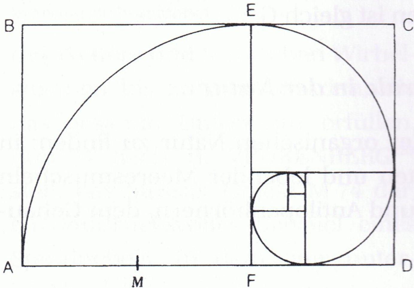
Abb. 32: Wirbelnde goldene Rechtecke erzeugen die goldene Spirale.
